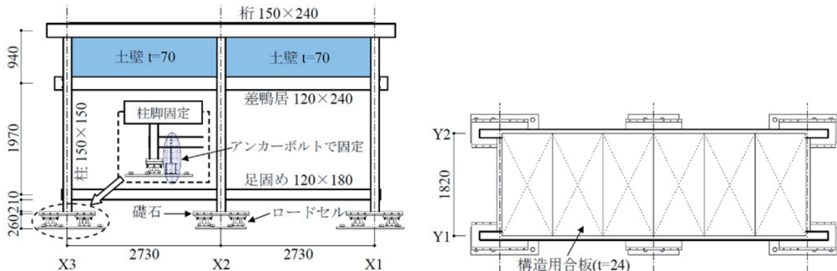
試験体図 (左：立面図、右：天井伏図)
